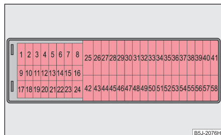
Obr. 204 Schématické zobrazení pojistkového boxu pro levostranné řízení
