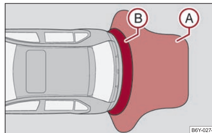
Obr. 126 Pomoc při parkování: dosah snímačů
