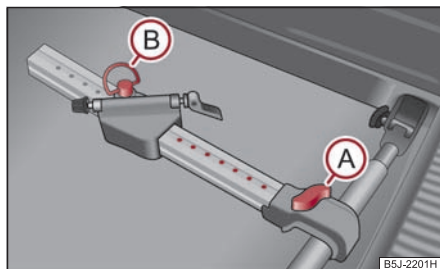
Obr. 92 Montáž držáku kol
