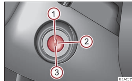
Obr. 123 Polohy klíče ve spínací skříňce
