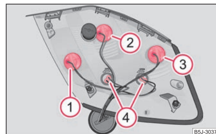
Obr. 218 Zadní skupinová svítilna: rozmístění žárovek
