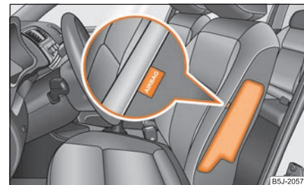
Obr. 152 Sedadlo řidiče: umístění airbagu
