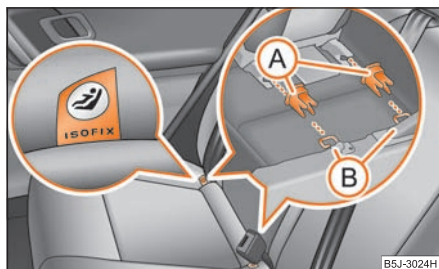
Obr. 165 Upevňovací oka (systém ISOFIX)
