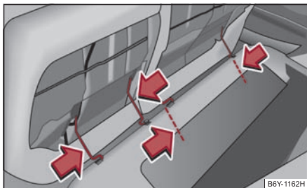
Obr. 70 Vyjmutí sedáku
