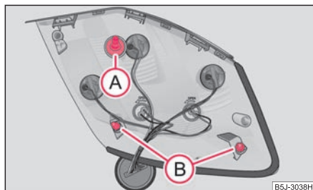
Obr. 217 Montáž zadní skupinové svítilny
