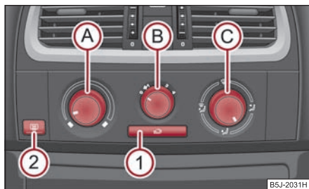
Obr. 118 Topení: ovládací prvky
