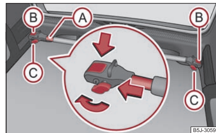
Obr. 91 Montáž příčniku
