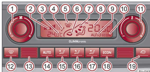
Obr. 120 Climatronic: ovládací prvky
