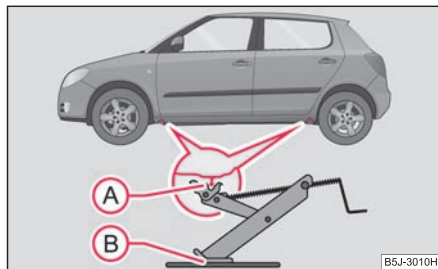
Obr. 197 Výměna kola: body pro nasazení zvedáku
