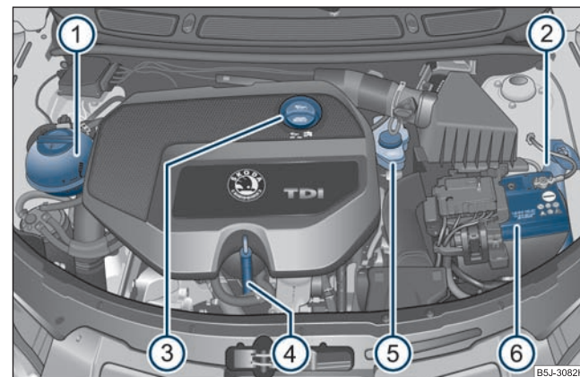
Obr. 181 Vznětový motor 1,9 l/77 kW
