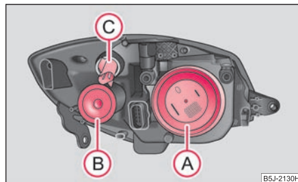
Obr. 211 Přední světlomet: rozmístění žárovek
