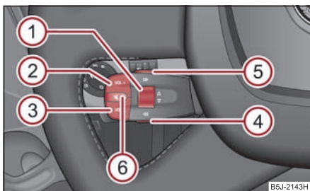
Obr. 132 Multifunkční modul: ovládací tlačítka autorádia
