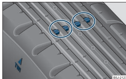
Obr. 190 Dežénové drážky pneumatiky s ukazateli opotřebení
