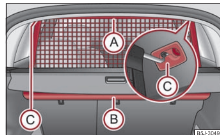
Obr. 86 Vytažení síťové mezistěny
